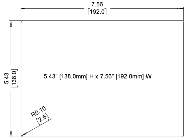
Cutout Dimensions
